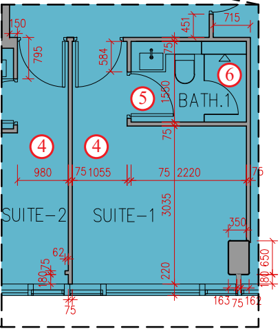
8/F Part Plan 8樓部份平面圖
